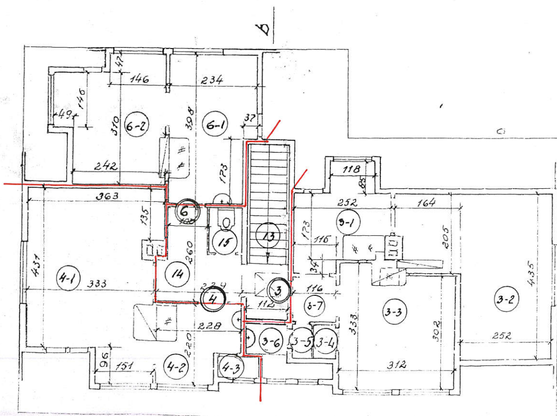
KATUSEKORRUS
