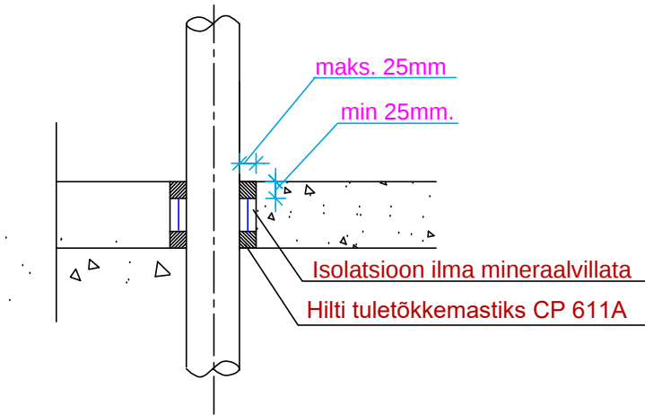
KÜTTETORU LÄBIVIHK PÕRANDAST (LAEST)
