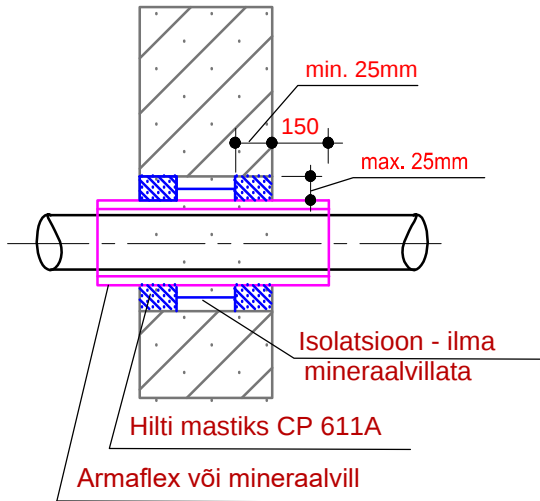
KÜTTETORU LÄBIVIHK TULETÕKKETARINDIST
