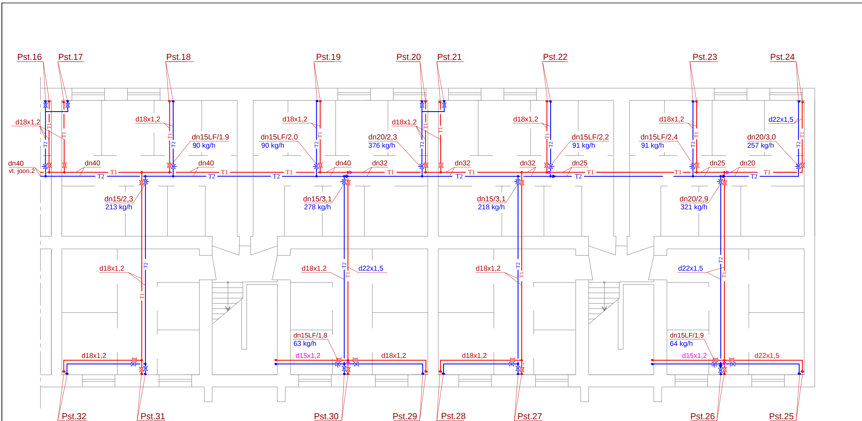
KÜTTETORU LÄBIVIHK PÕRANDAST (LAEST)
